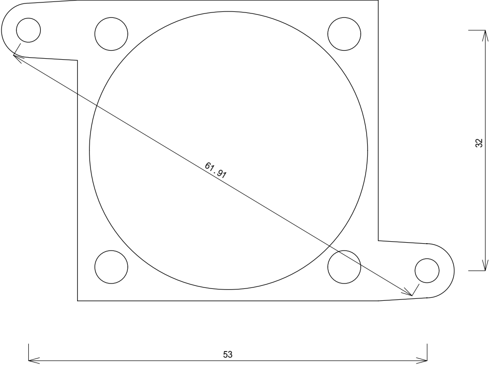
ASUS P5Q Steel shield
